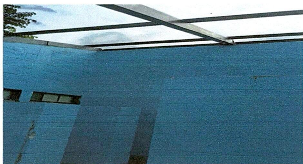
Foto 3: Acá nos muestra la instalacion de techo renovado para la colocación servicios de cableado y la de accesorios eléctricos para la iluminación de los servicios sanitarios.
